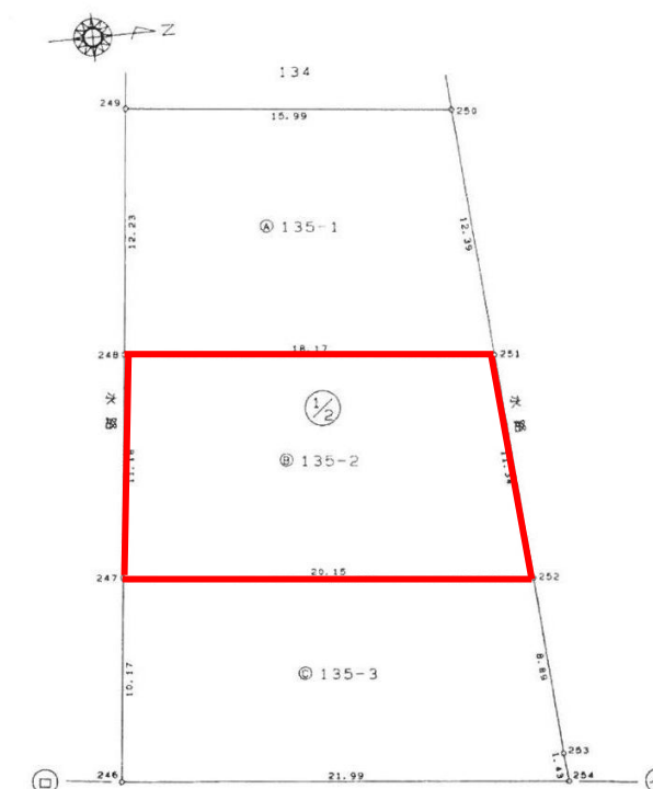
測量図
